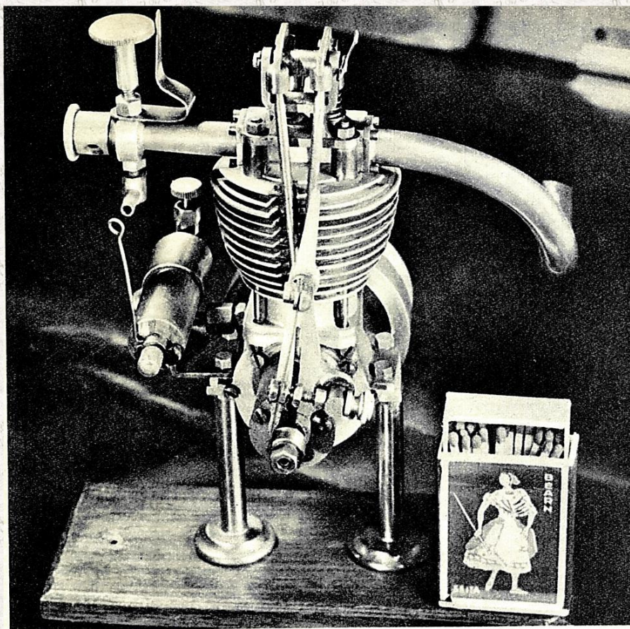
Ce monocylindre à 4 temps développe 0,700 ch à 4200 t/m.
